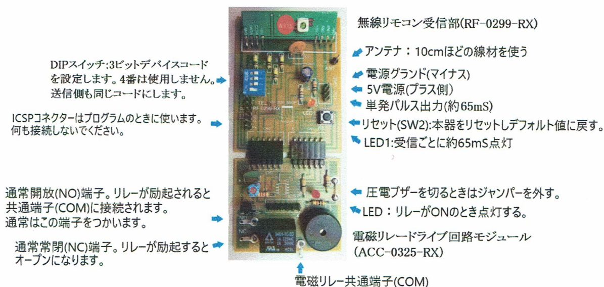
電磁リレードライブ回路モジュール(ACC-0325-RX)を使った 315メガ帯RFリモコン受信機 品番RF-0299-RX-RR
