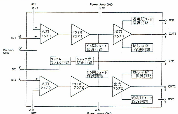
等価回路ブロック図
